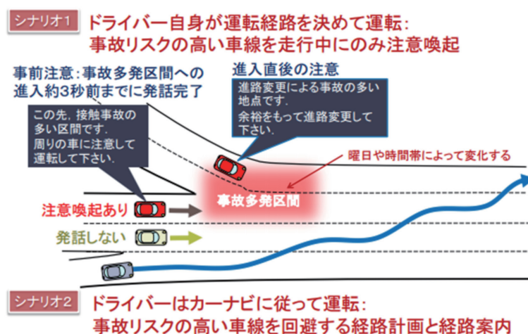
図 13-1 カーナビによる安全運転支援情報の提供（シナリオ別）
