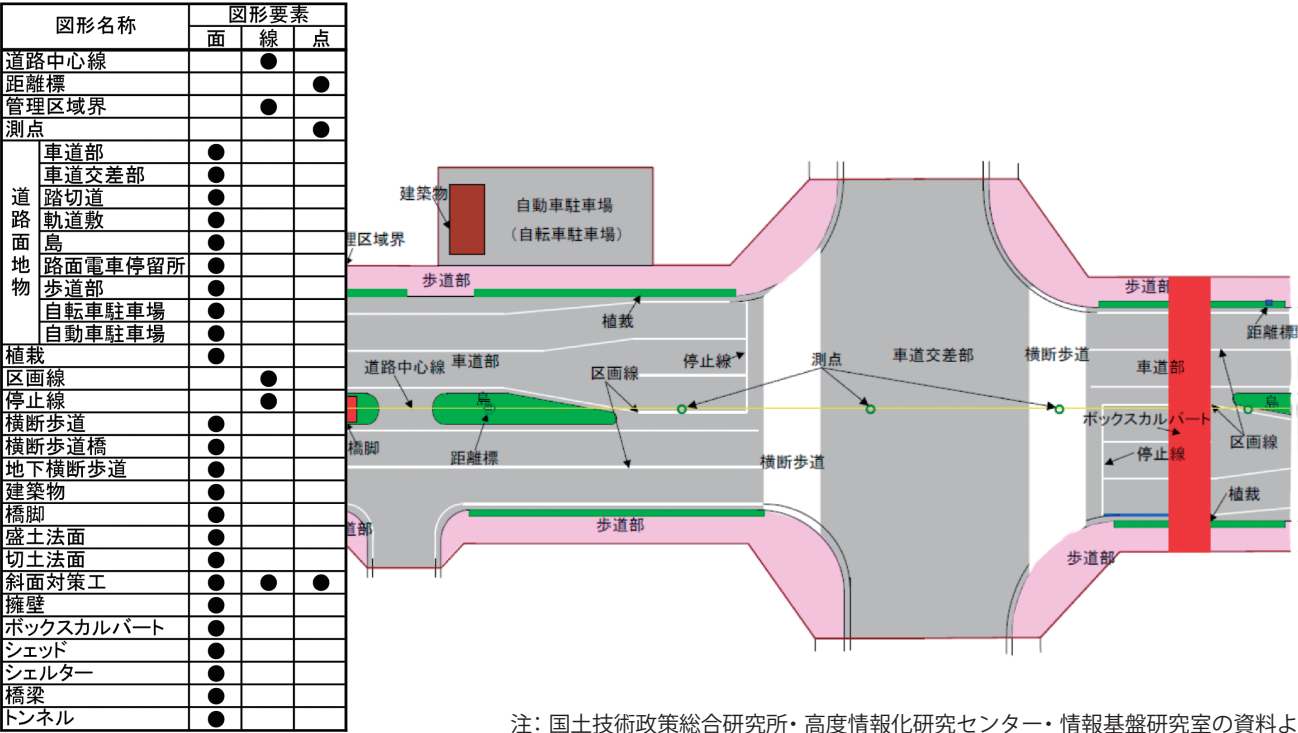
図 12-2 道路基盤地図情報のイメージ
