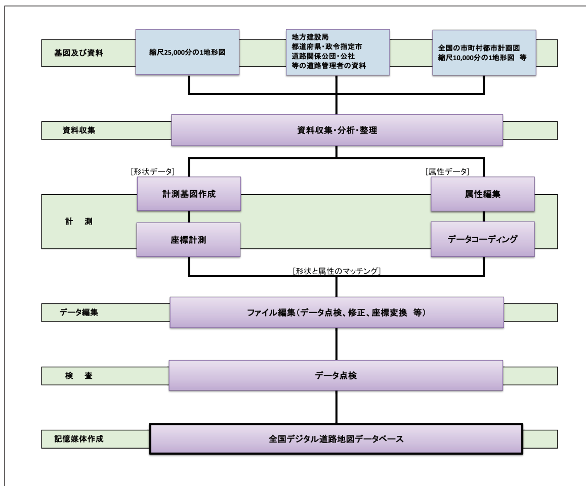
図 3-5 標準的な全国デジタル道路地図データベースの作成フロー
