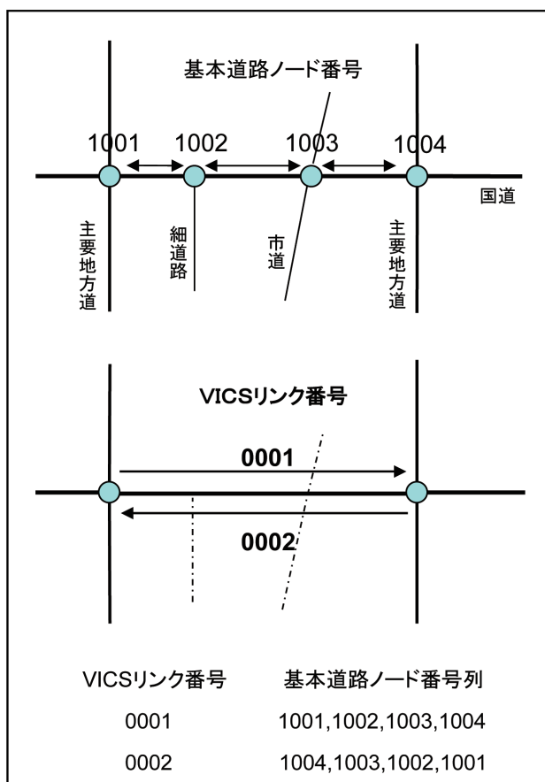
図 6-2 VICS リンク番号
