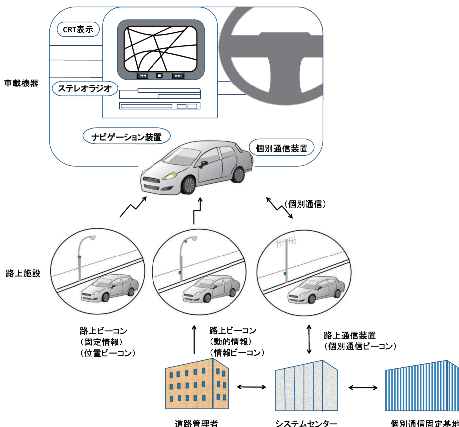
図 2-1 路車間情報システムのイメージ
