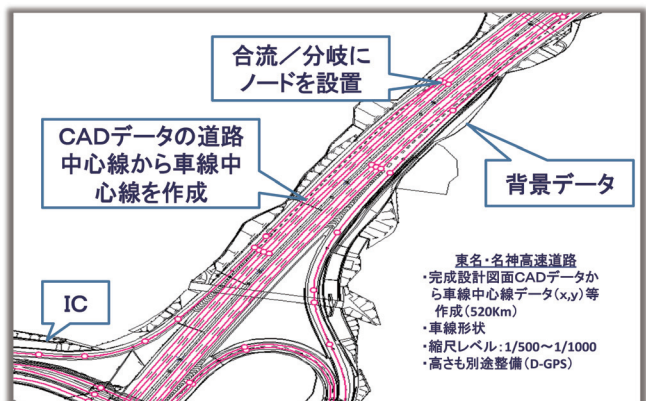
図 11-3 高速道路の高度 DRM-DB
